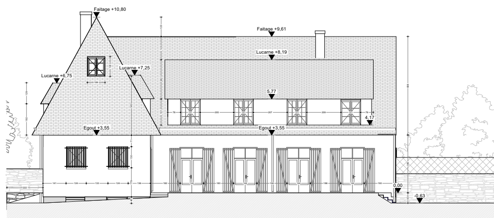
Élévation façade Sud existante - phase relevé
