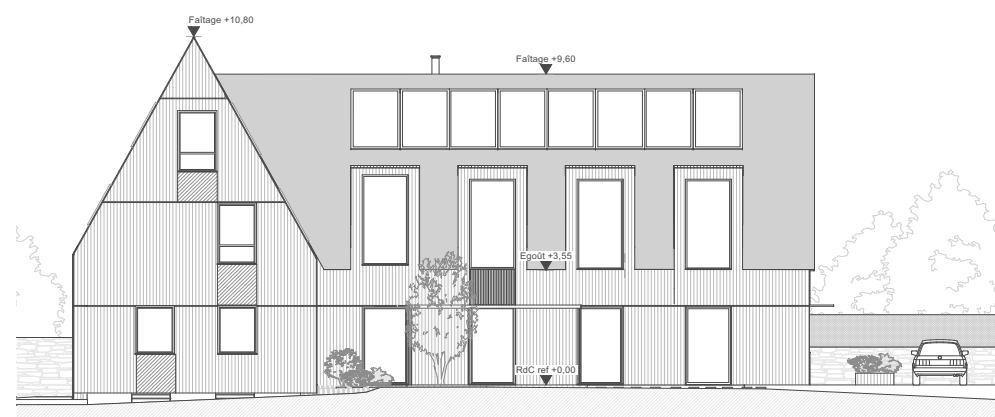
Élévation façade Sud projet - phase esquisse
