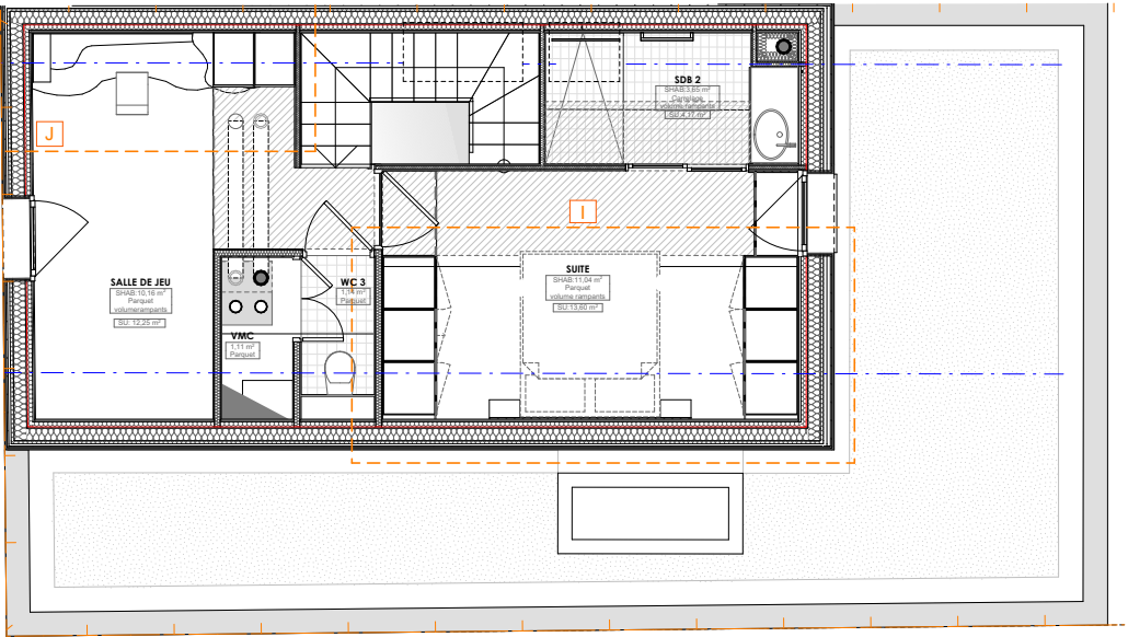
Plan R+2
