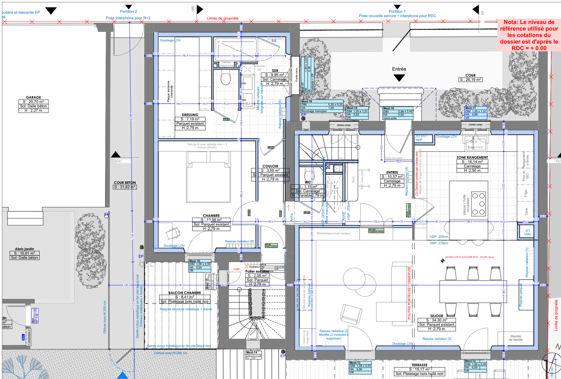
Plan RDC projet - phase DCE
