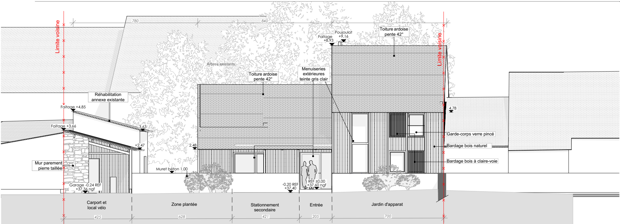
Façade Est - phase PC
