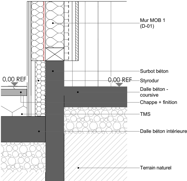
Détail pied de mur
