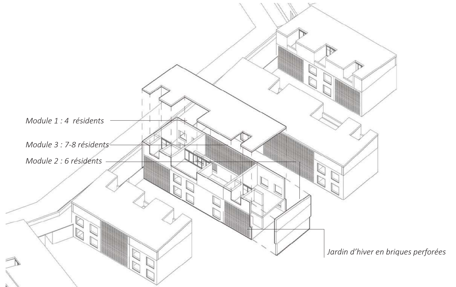
Axonométrie répartition des logements
