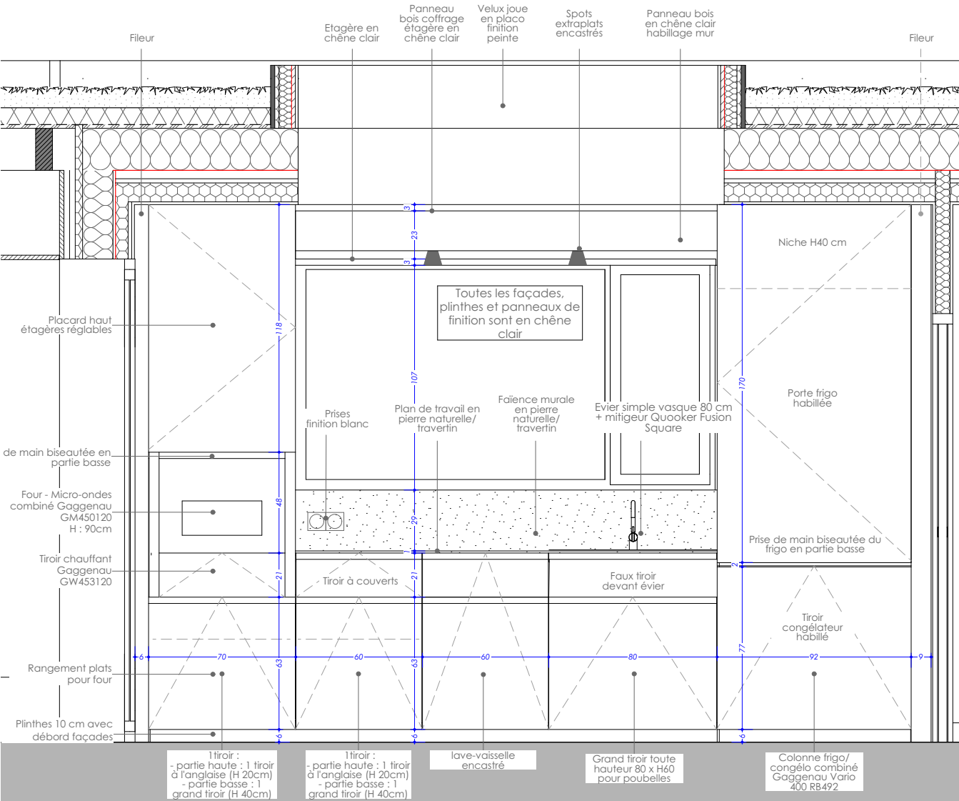
Elévation cuisine 1/20
