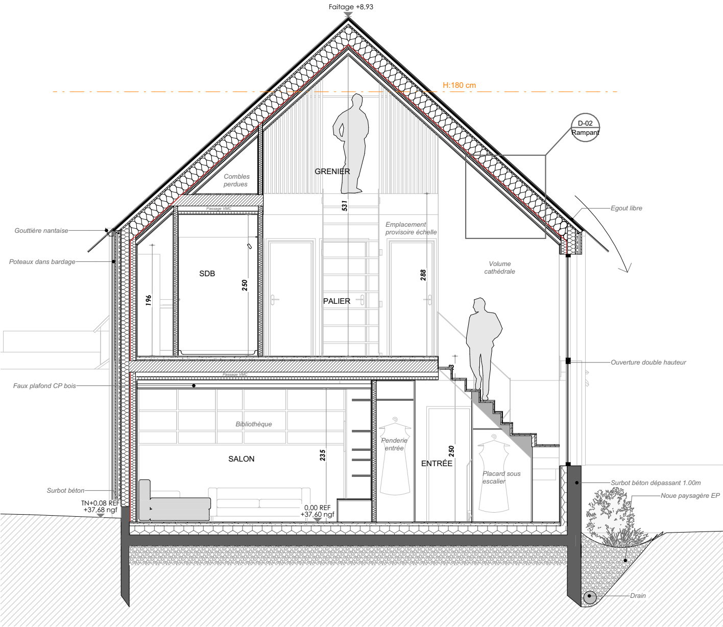
Coupe détaillée - phase APD
