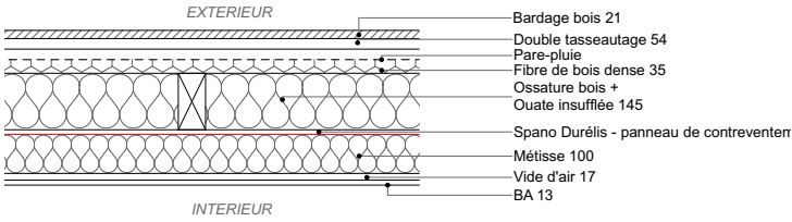
Détail mur périphérique à ossature bois
