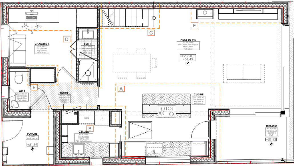
Plan RDC
