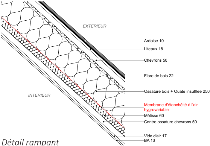
Détail rampant
