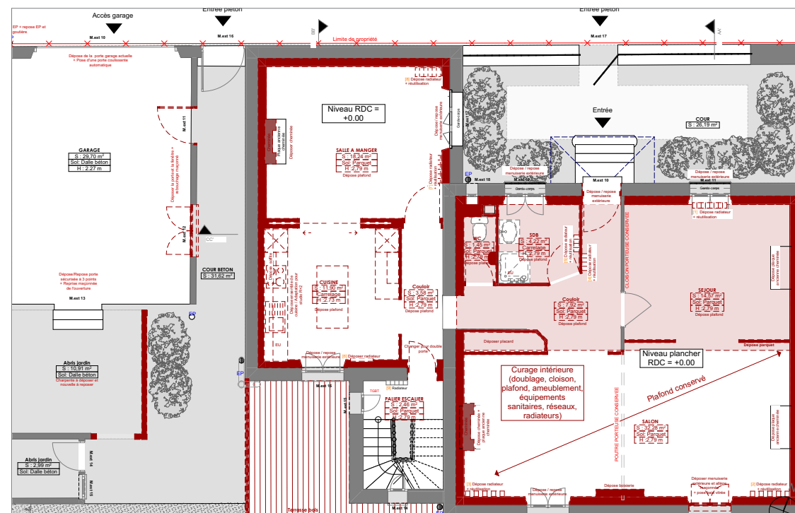
Plan RDC démolition - phase DCE
