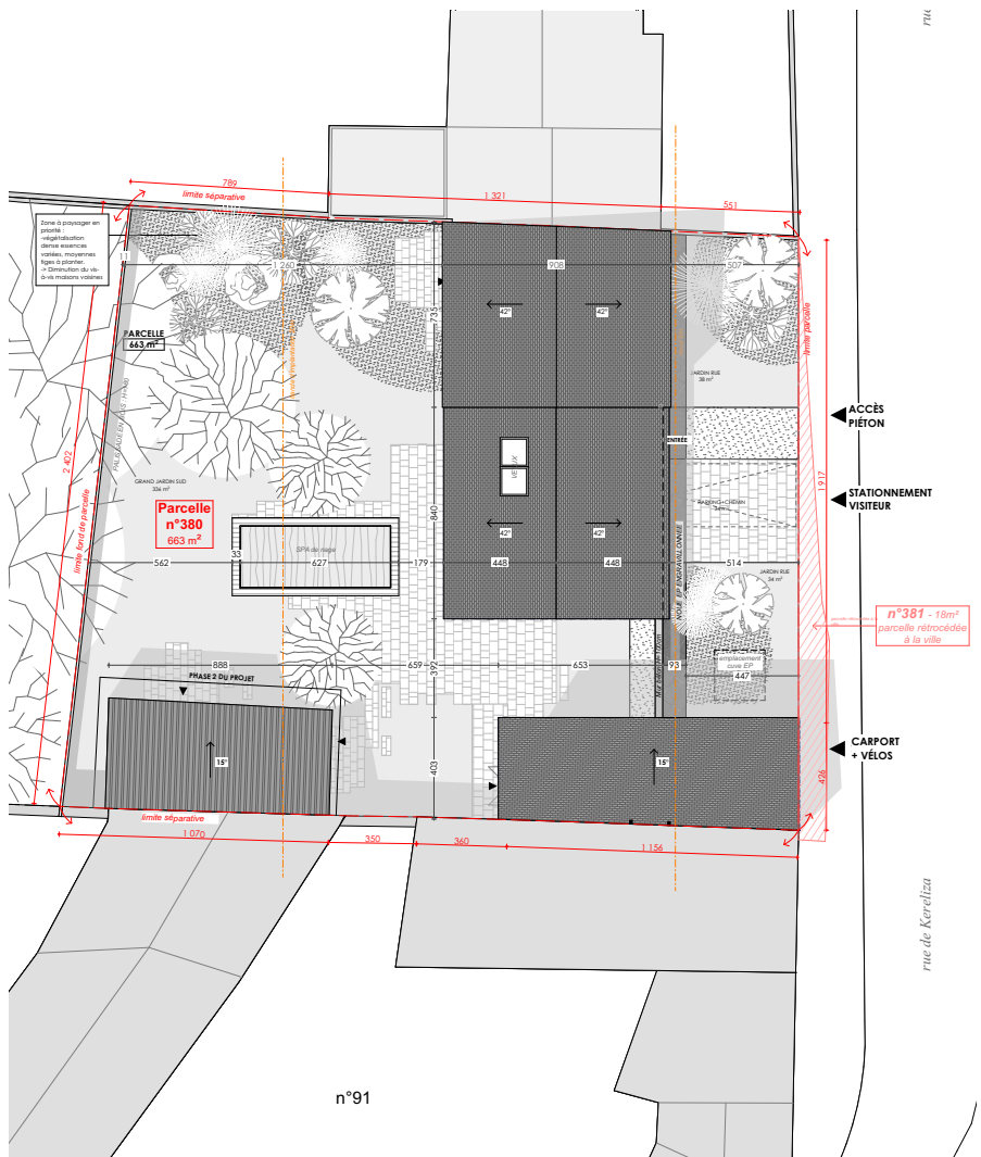
🕒 Plan masse - phase APS
