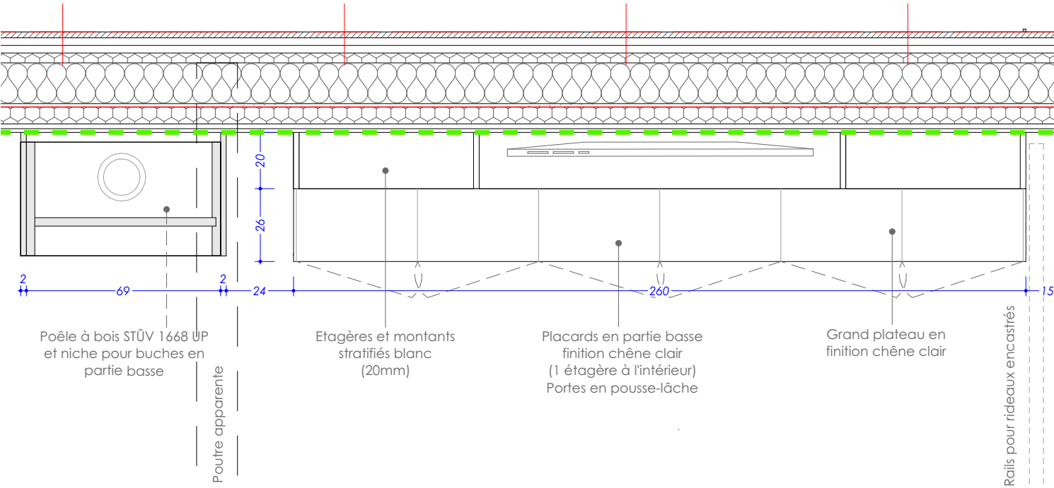
Plan agencement salon 1/20
